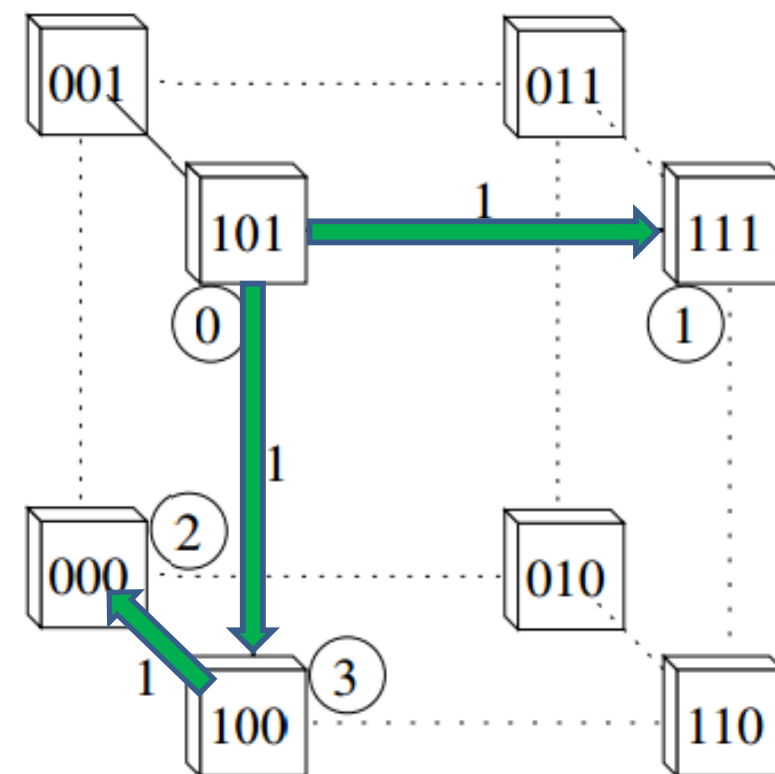
(d) Mapping \Gamma_2 .
